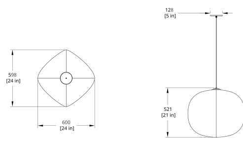
MP-S Mori Squash Pendant Dimension
